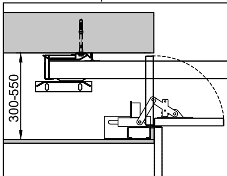
Seitenklappe "optional"
