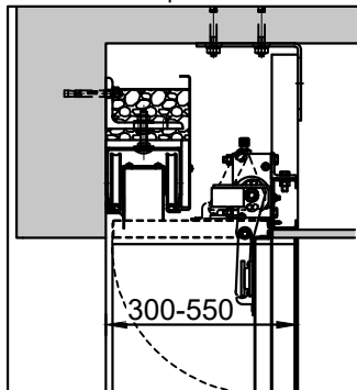
Deckenklappe "optional"
